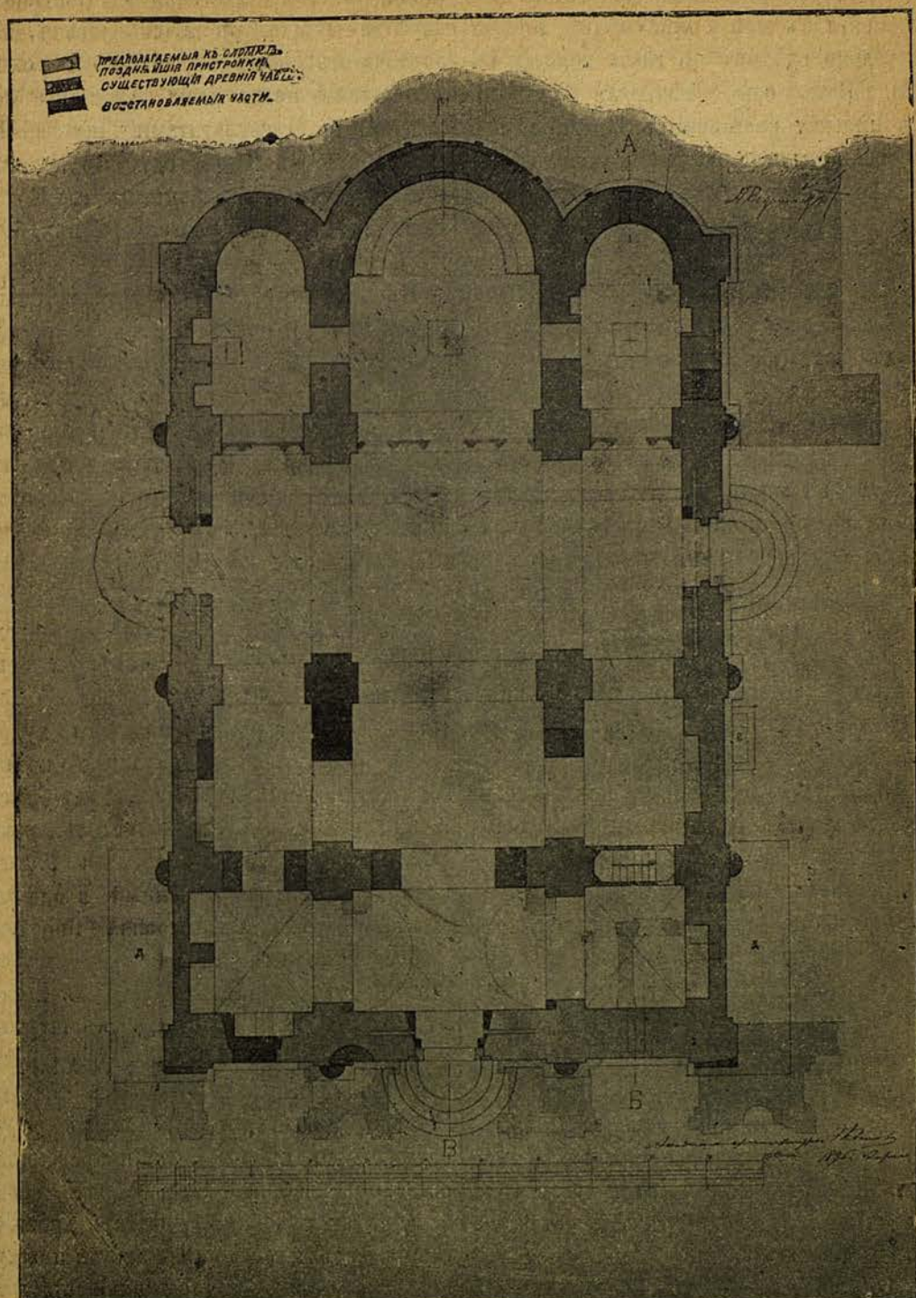
Планъ Мстиславова храма въ его первоначальныхъ очертаніяхъ.
