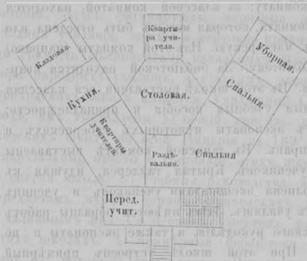
Планъ II-го этажа.
