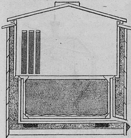
Американскій улей Рута.
