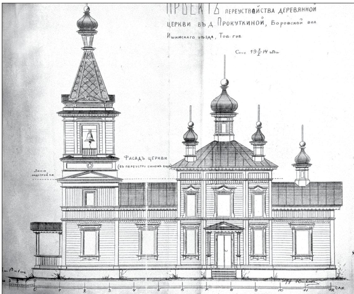
Фасад реконструируемой Христорождественской церкви из проекта архитектора Н. А. Юшкова. 2 января 1914 г. ГА в г. Тобольске.
