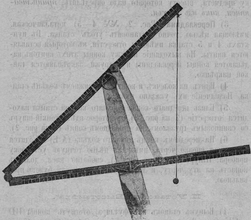
Рис. 1. Видъ Высотомѣра по фотографіи съ природы, при измѣреніи высоты. Нитка съ грузиломъ направо. Львѣе—перекладина цинковая, привинченная гайками. Еще львѣе—палка, къ которой прикрѣпленъ аппаратъ. На верху видно кольцо винта, коимъ аппаратъ привинченъ къ верхнему концу палки. Внизу виденъ узелъ веревки, которою аппаратъ привязанъ къ палкѣ. Палка взята самая обыкновенная и обтесана топоромъ. Весь приборъ можно носить вмѣсто трости.
