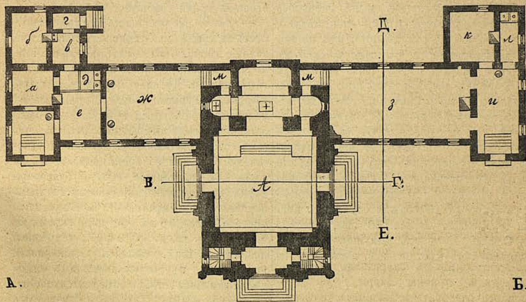
Планъ церкви-школы.
