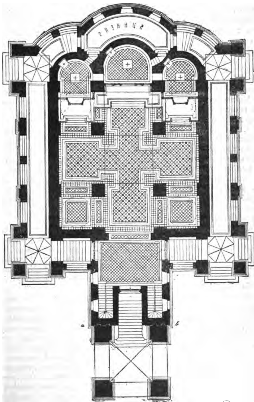
Планъ храма у подножія Балкана.
