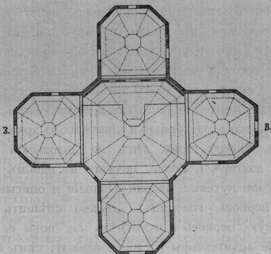
Рис. 13 и 14. Разрѣзъ и планъ церкви м. Ярышева.
