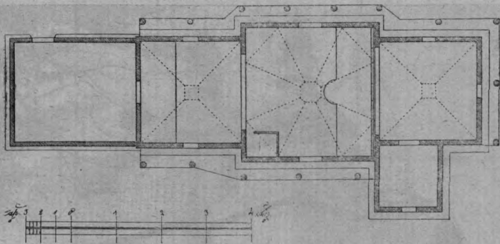
Рис. 4. Планъ церкви с. Старыхъ Хуторовъ.
