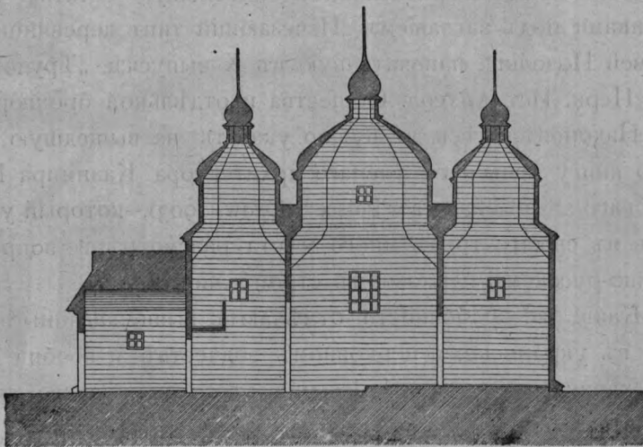
Рис. 7. Разрѣзъ церкви с. Малыхъ Хуторовъ.
