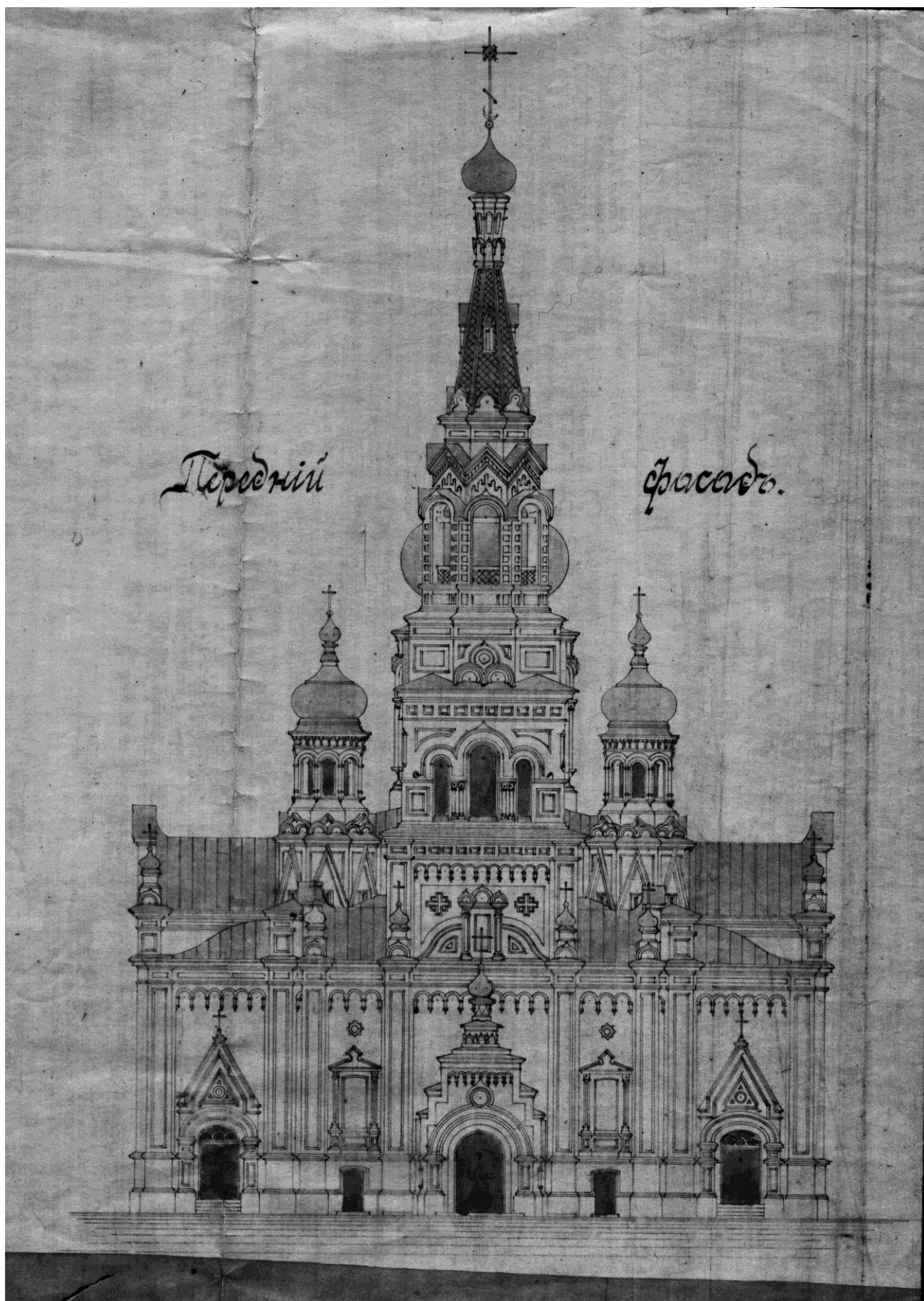
Лист переднего фасада храма из дела «Об утверждении проекта каменного храма в селе Виловатом Бузулукского уезда». 1900 г.
