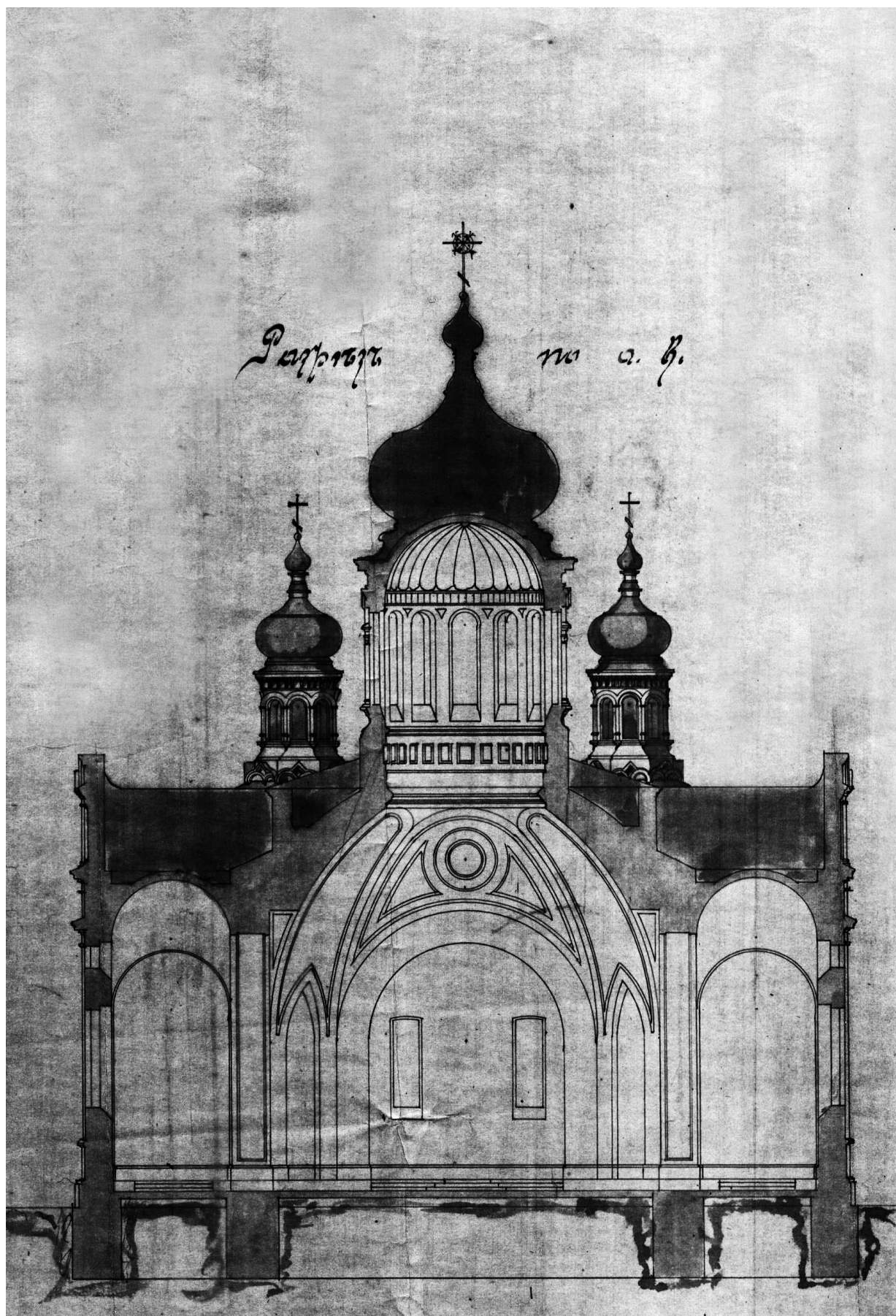
Фронтальный разрез храма из дела «Об утверждении проекта каменного храма в селе Виловатом Бузулукского уезда». 1900 г.
