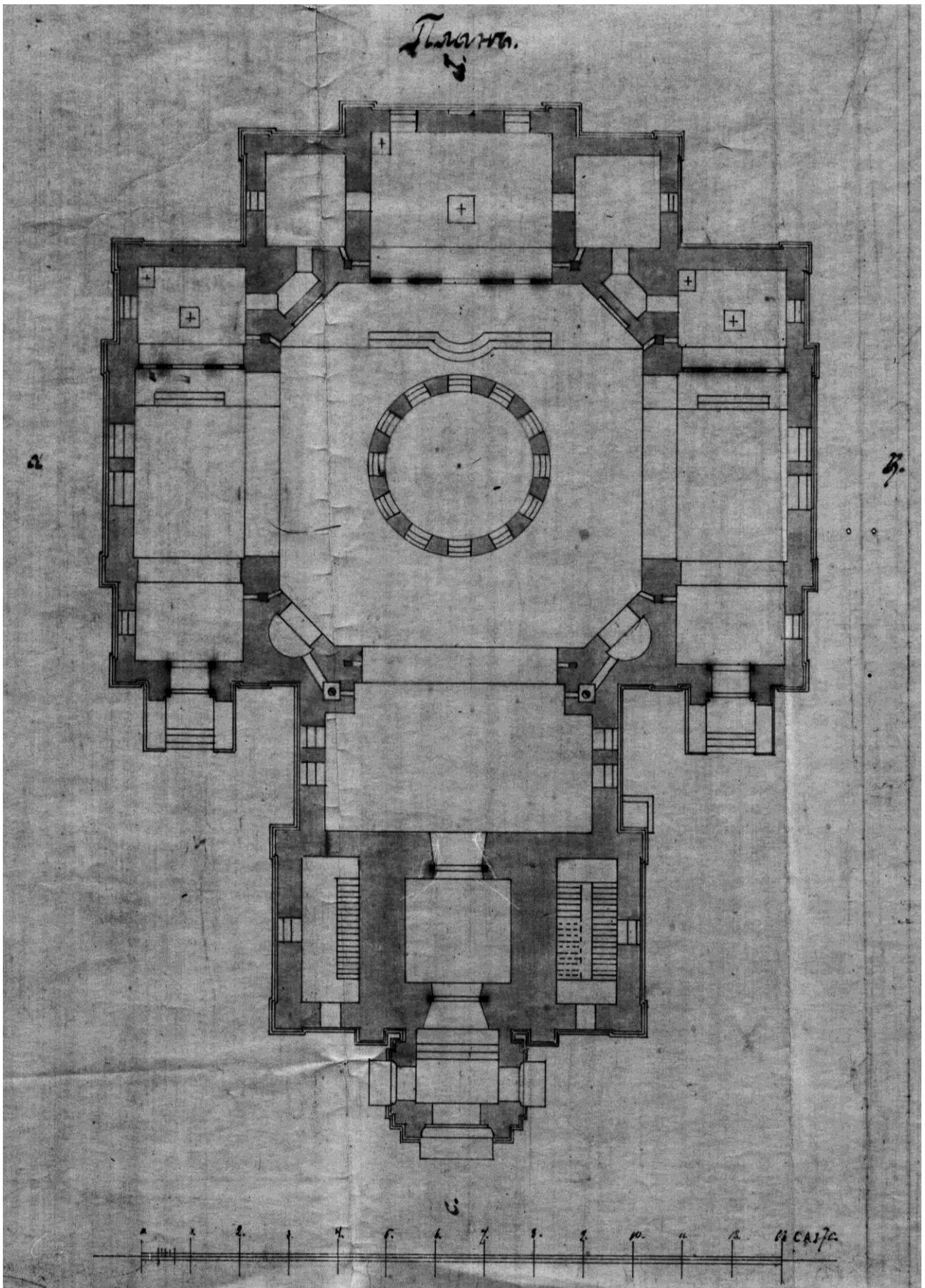
План храма из дела «Об утверждении проекта каменного храма в селе Виловатом Бузулукского уезда». 1900 г.
