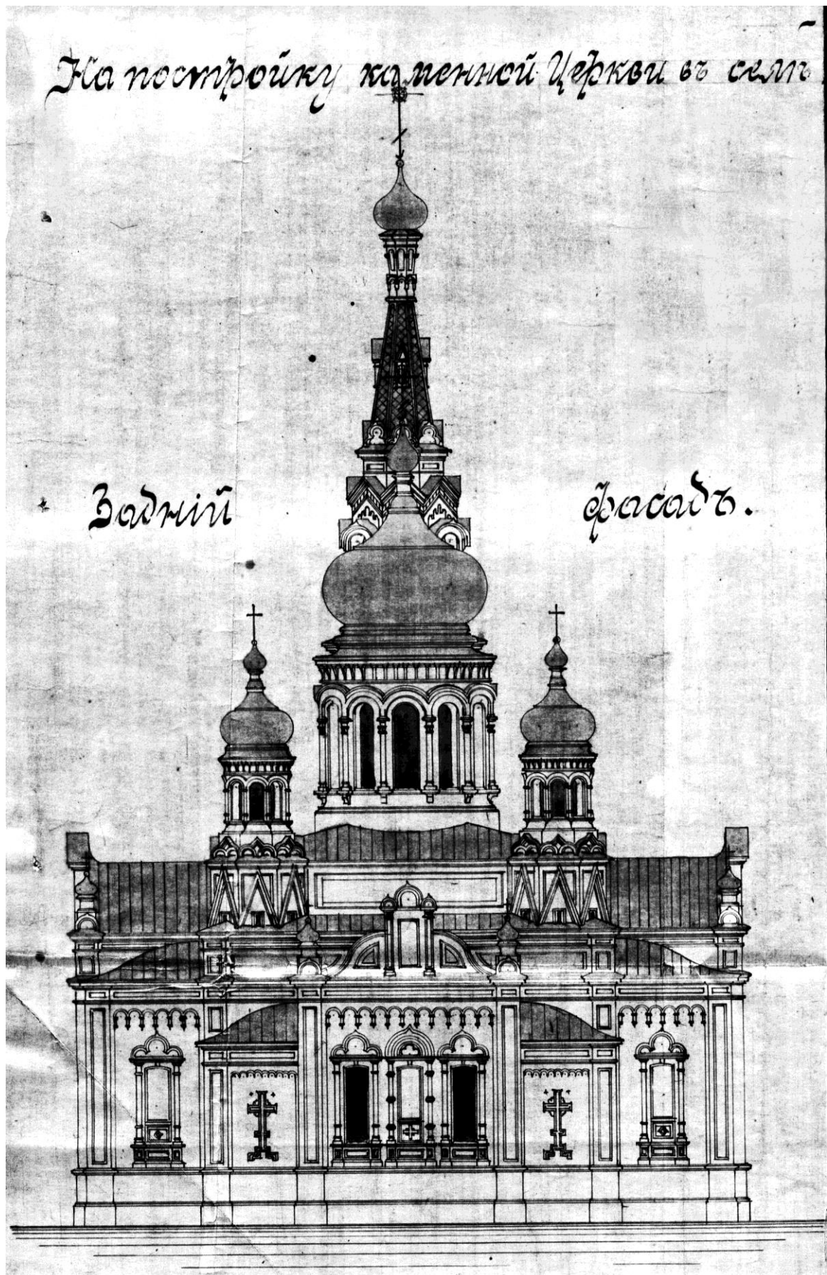
Лист заднего фасада храма из дела «Об утверждении проекта каменного храма в селе Виловатом Бузулукского уезда». 1900 г.
