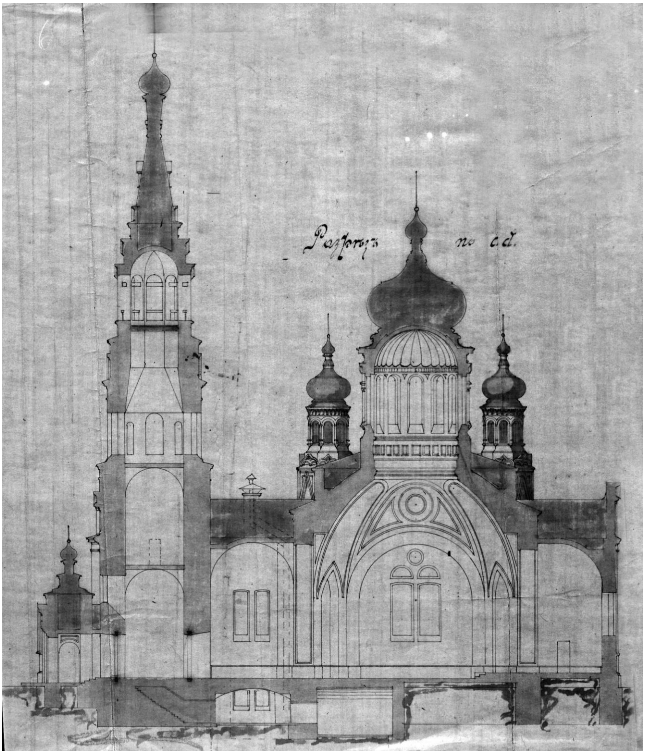
Боковой разрез храма из Дела «Об утверждении проекта каменного храма в селе Виловатом Бузулукского уезда». 1900 г.
